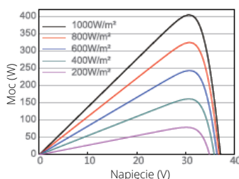
Krzywa Moc - Napięcie JAM54S30-405/MR
