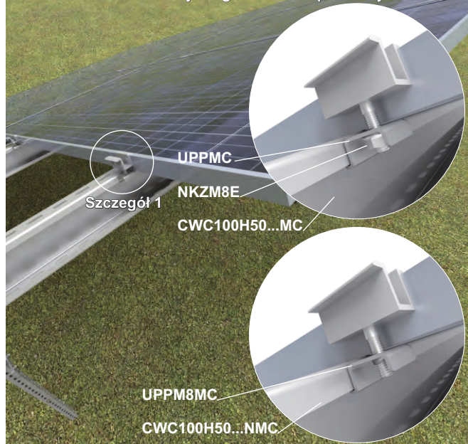
Montaż pośredniego uchwyty UPPMC do ceownika CWC100H50...MC w miejscu gdzie nie ma perforacji
