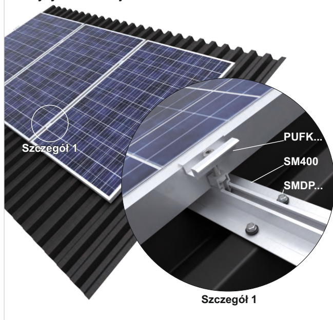
Montaż pośredniego uchwyty klik PUFK do szyny aluminiowej SM400
