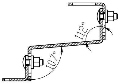
PRZEKRÓJ A-A SKALA 1 : 4
